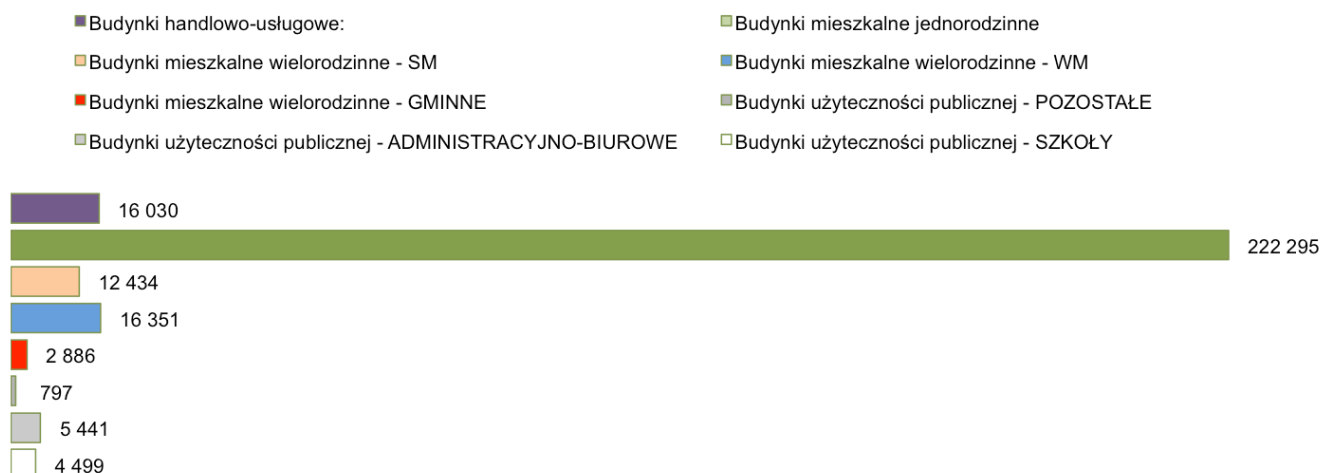
Wykres 5.2.5-1 Zużycie energii finalnej w budownictwie w roku bazowym 2013 [MWh/rok]
