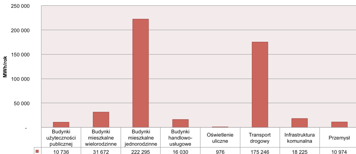
Wykres 2.2.1-1 Zużycie energii finalnej na obszarze gminy Żnin w roku bazowym 2013
